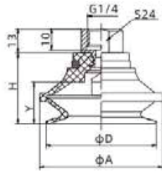
SZB50□-G2F
