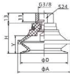
SZB50□-G3F
